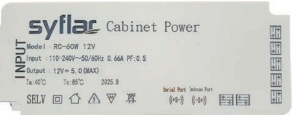
FONTE GABINETE 60W
